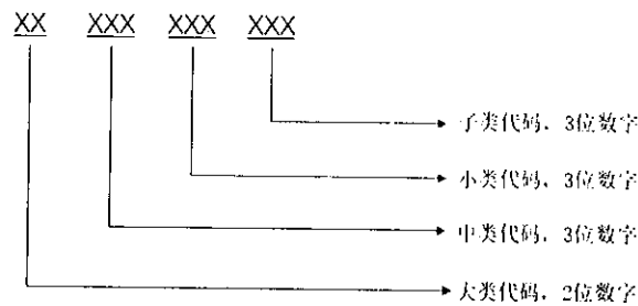
图 4 农业信息数据编码代码结构图
